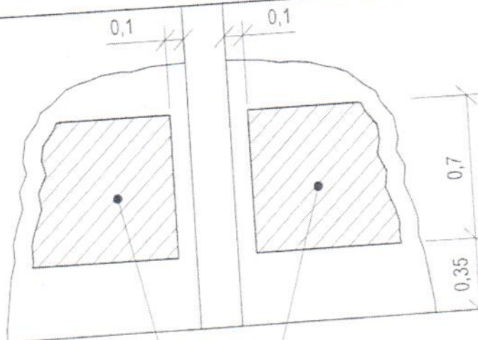
1 Pomnik - wymiary 1:50
